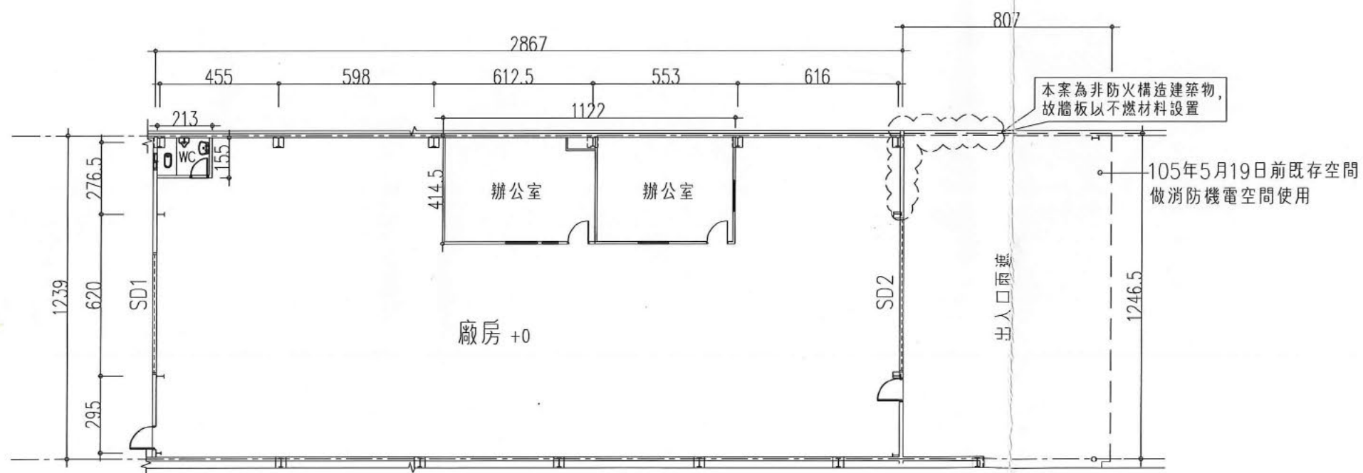
壹層平面圖 A1: S=1/100 A3: S=1/200
